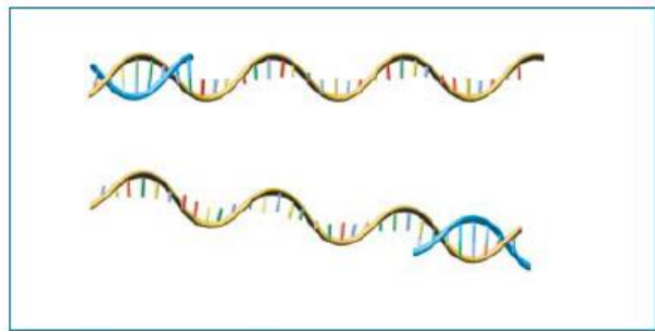
Paso 2: Annealing
