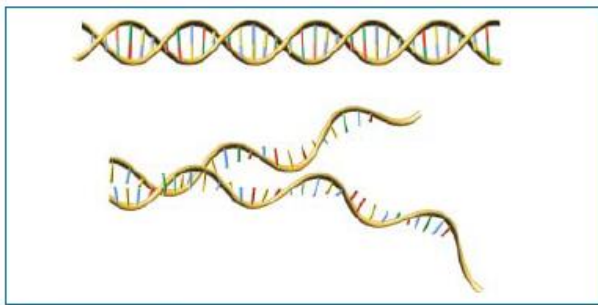
Paso 1: Desnaturalización
